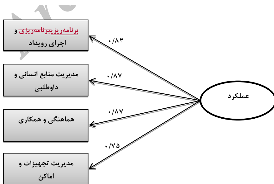
شکل ۳. مدل تحلیل عاملی مرتبه دوم عملکرد در انجمن‌های ورزشی در حالت تخمین استاندارد
