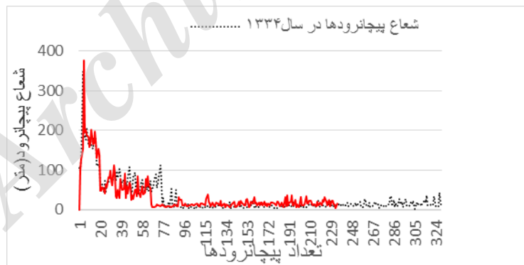
شکل (۹) تغییرات شعاع پيچانرودهای رودخانهی قره سو
