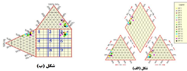
شکل (۷) نمودارهای پایپر (لف) و دورو (ب) برای نمونه‌های آب زیرزمینی منطقه
