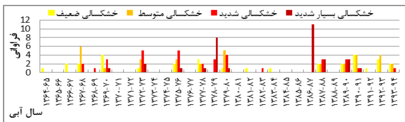
شکل (۲) فراوانی خشک‌سالی هواشناسی بر اساس شاخص DI در حوضه‌ی آبخیز کارون شمالی، (۹۴-۱۳۶۴)
