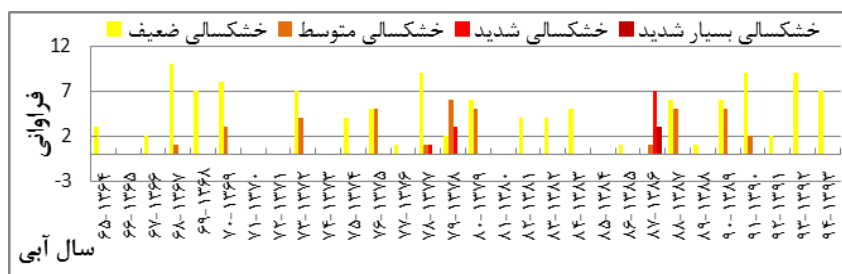
شکل (۳) فراوانی خشک‌سالی هواشناسی بر اساس شاخص Z score در حوضه‌ی آبخیز کارون شمالی (۹۴-۱۳۶۴)
