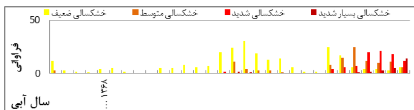
شکل (۶) فراوانی خشک‌سالی هیدروژئولوژیکی بر اساس GRI در حوضه‌ی آبخیز کارون شمالی (۹۴-۱۳۶۴)
