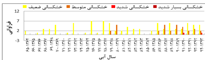
شکل (۴) فراوانی خشک‌سالی هیدروژئولوژیکی بر اساس شاخص SDI در حوضه‌ی آبخیز کارون شمالی (۱۳۶۴-۹۴)
