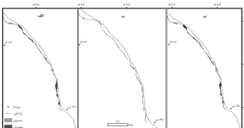
شکل (۷) (بالا) پهنه‌های پیشروی و پسروی کناره‌ی راست (بالا) و پهنه‌های پیشروی و پسروی چپ (پایین) دوره‌ی اول (الف)، دوره‌ی دوم (ب) و دوره‌ی سوم (پ)
