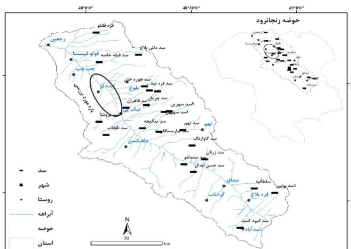
شکل (۶) موقعیت سد‌های حادث شده در حوضه‌ی زنجانرود
