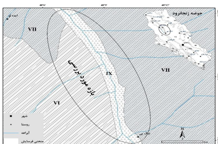
شکل (۵) طبقات فرسایش محدوده‌ی مورد مطالعه
