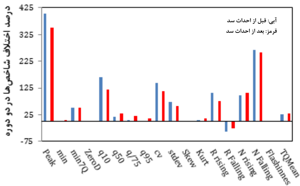
شکل (۱۴) هیستوگرام مقادیر شاخص‌های هیدرولوژیک در دوره‌های قبل و بعد از احداث سد در ایستگاه هیدرومتری ساری‌قامیش
