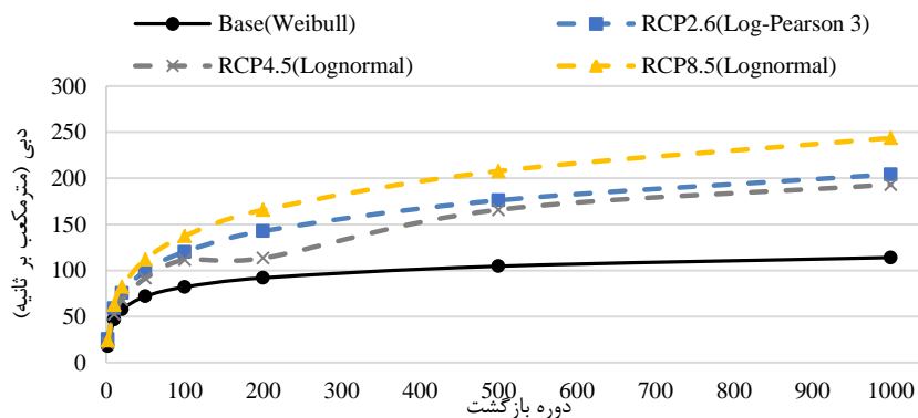
شکل (۵) مقایسه تغییرات شدت دبی‌های پیک در دوره پایه و آتی در دوره بازگشت‌های ثابت Fig (5) Comparison of changes in peak discharge at constant return periods for the base and future periods
