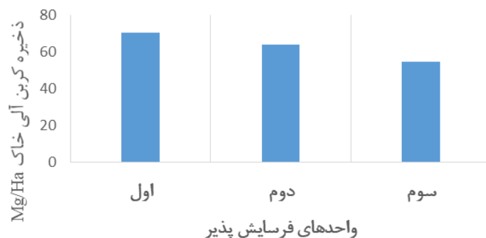
شکل (۸) میزان ذخیره کربن آلی در واحدهای مختلف فرسایش‌پذیر Fig (8) Organic carbon storage in different erodible units
