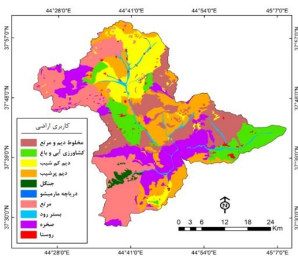
شکل (۴): نقشه‌ی کاربری اراضی Fig (4): Landuse map
