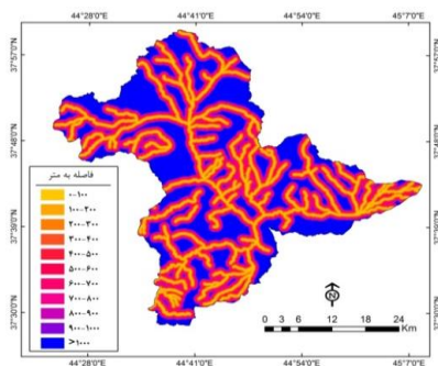
شکل (۶): نقشه‌ی فاصله از آبراهه Fig (6): Distance to stream map
