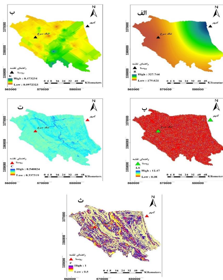
شکل (۳): نقشه پارامترهای مدل RUSLE در حوضه آبریز تنگ سرخ: (الف) شاخص فرسایندهی باران (R)، (ب) شاخص فرسایش پذیری خاک (K)، (پ) شاخص LS، (ت) شاخص پوشش گیاهی (C)، (ث) شاخص عملیات حفاظت خاک (P)
