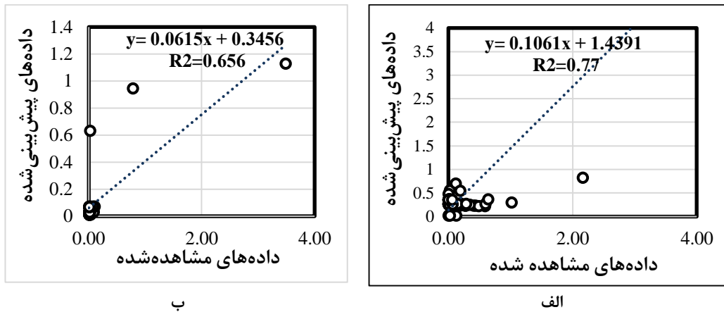
شکل (4): همبستگی داده‌های رواناب مشاهده‌شده و پیش‌بینی‌شده مدل در مرحله الف) واسنجی و ب) اعتبارسنجی در ایستگاه کوزه‌تیراقي
