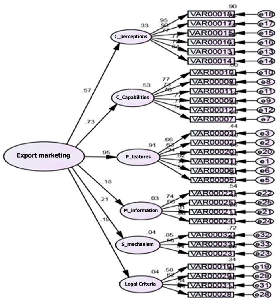
شکل (۱). تحلیل عاملی اکتشافی مدل کلی پژوهش با ضرایب استاندارد
