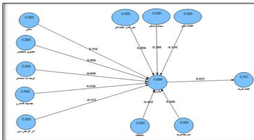
شکل ۴) ضرایب مسیر
