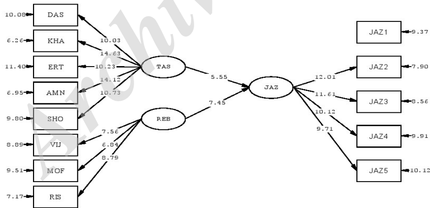
شکل ۲. آزمون تحلیل مسیر برای فرضیه‌های اول و دوم پژوهش
