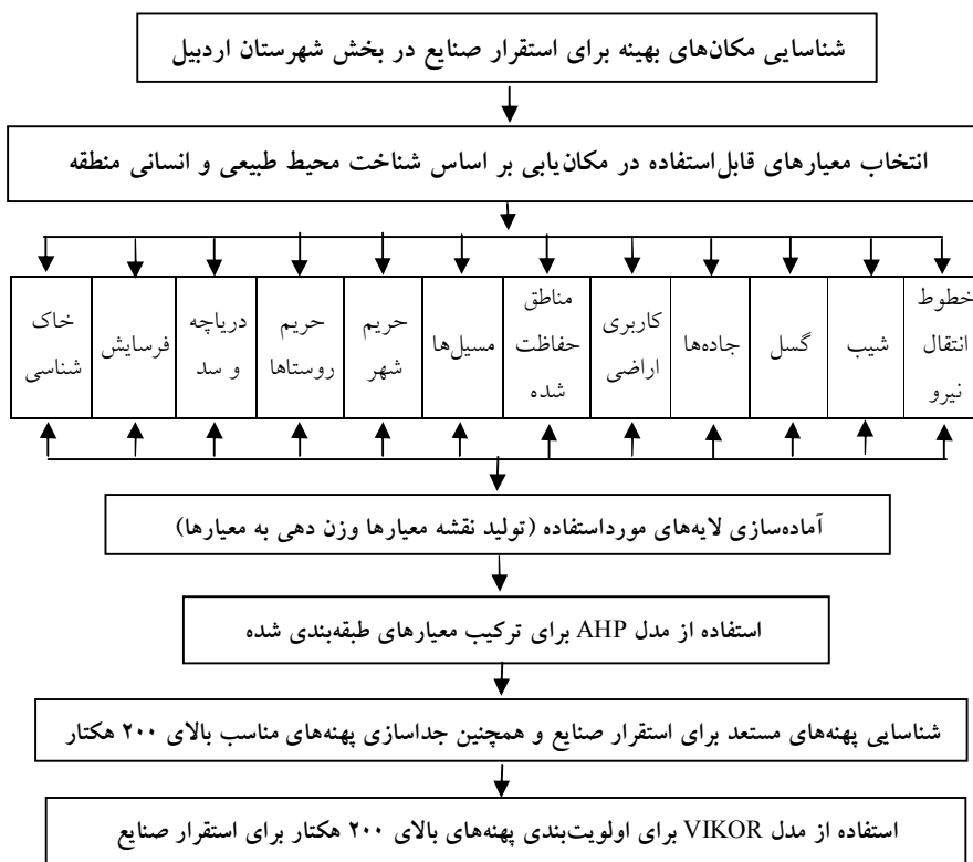
شکل ۱- فلوچارت روند کلی مکان‌یابی صنعتی در شهرستان اردبیل
