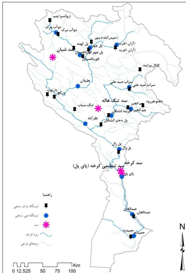
شکل ۱- موقعیت ایستگاه‌های هیدرومتریک، باران‌سنجی و سد‌های حوضه آبریز کرخه
