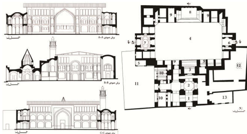
تصویر (۷): پلان و برش‌های وضع موجود بقعه پنجه‌شاه (نگارندگان: بر اساس گنجنامه)
