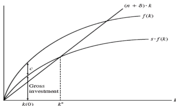
نمودار شماره ۱: مدل سوان - سولو
