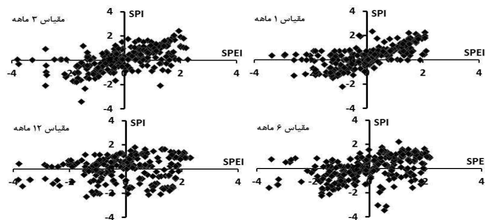
شکل ۲: ارتباط بین شاخص‌های خشکسالی SPI و SPEI
