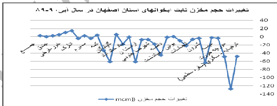
شکل ۴: نمودار تغییرات حجم مخزن ثابت آبخوانهای استان اصفهان در سال آبی ۱۳۸۹-۹۰
