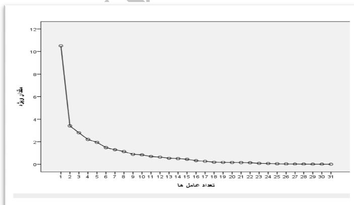
شکل ۲. نمودار سنگریزه‌ای برای تعیین تعداد عامل‌ها
