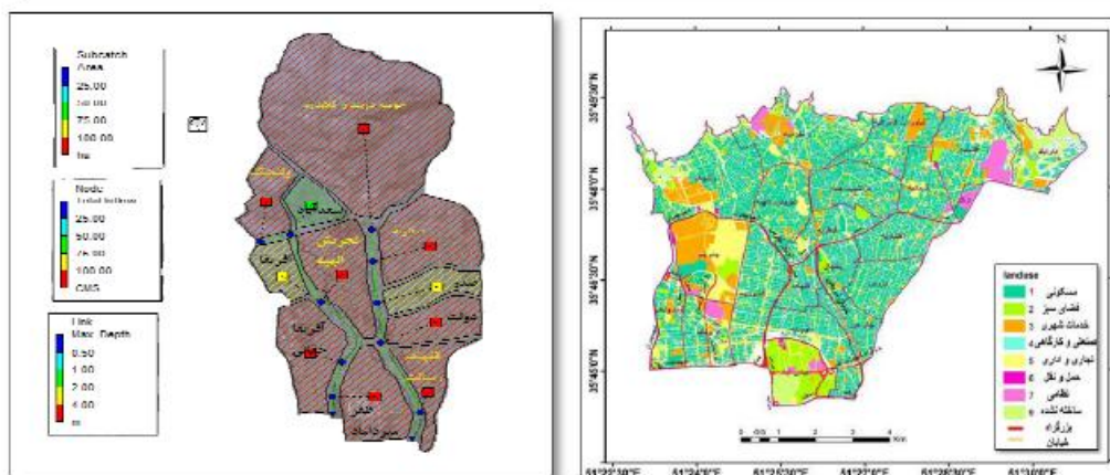
شکل ۵: شماتیک حوضه‌بندی و زهکش منطقه در نرم‌افزار SWMM
