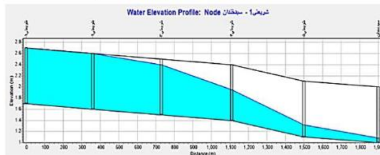
شکل ۸: پروفیل طولی خیابان شریعتی
