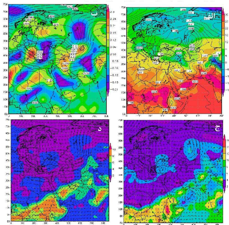
شکل ۳. الف: ترکیبی دما و فشار تراز دریا، ب: ترکیبی ارتفاع ژئوپتانسیل و امگای تراز ۷۰۰ هکتوپاسکال، ج و د: ترکیبی رطوبت و بردار باد در ترازهای ۸۵۰ و ۷۰۰ هکتوپاسکال روز ۲۵ فروردین ۱۳۹۰
