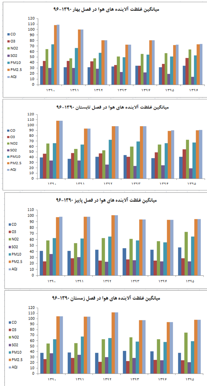
شکل ۲: نمودار میانگین فصلی غلظت آلاینده‌های ایستگاههای منطقه پژوهش در دوره ۱۳۹۰ تا ۱۳۹۶
