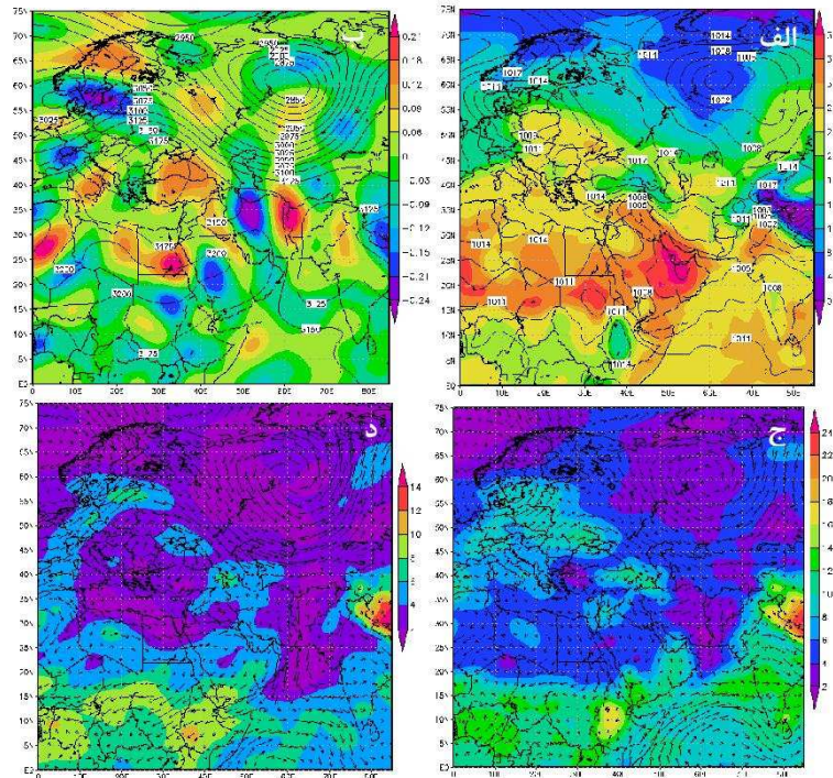
شکل ۴. الف: ترکیبی دما و فشار تراز دریا، ب: ترکیبی ارتفاع ژئوپتانسیل و امگای تراز ۷۰۰ هکتوپاسکال، ج و د: ترکیبی رطوبت و بردار
