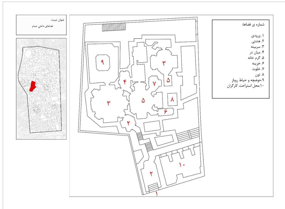
تصویر ۱: تقسیم‌بندی فضاهای داخلی حمام محتشم کاشان
