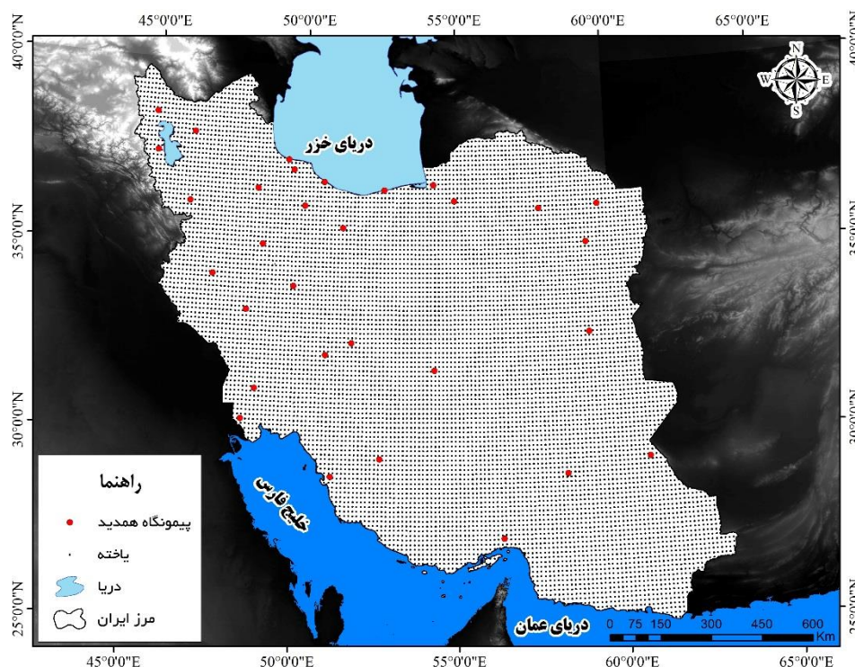
شکل ۱: پایگاه داده مرکز پیش‌بینی میان‌مدت هواسپهر اروپایی (ECMWF) نسخه ERA-Interim با تفکیک مکانی ۰/۱۲۵×۰/۱۲۵ درجه قوسی به همراه پیمونگه‌های همدید شاخص
