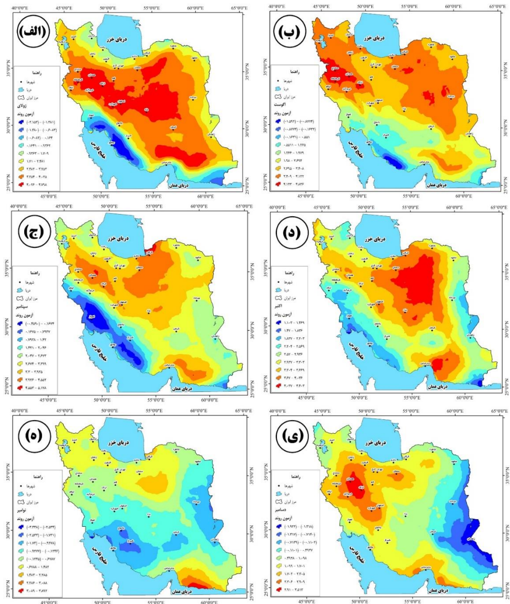
شکل ۳: روند دمای ایران مبتنی بر برونداد پایگاه داده پیش‌بینی میان‌مدت هواسپهر اروپایی (ECMWF) نسخه ERA Interim (الف: ژوئیه؛ ب: ماه آگوست؛ ج: ماه سپتامبر؛ د: ماه اکتبر؛ ه: ماه نوامبر؛ ی: ماه دسامبر)
