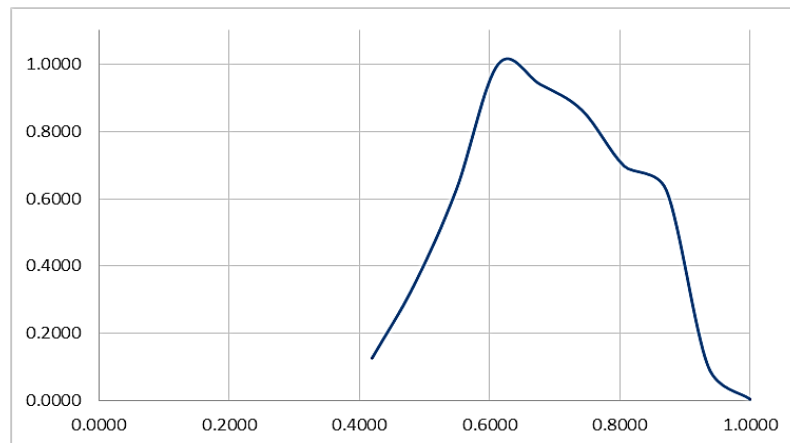
شکل ۷: منحنی انتگرال هیپسومتری حوضه آبریز ۸-۲-۲-۴ (ترسیم: نگارنده، ۱۳۹۷)
