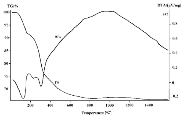
شکل (۳): نتایج آنالیز حرارتی همزمان ترکیب سرباره
