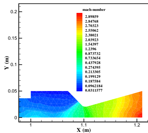
شکل ۹- کانتور عدد ماخ در ناحیه نازل در ثانیه سوم سوزش بدون فرسایش
