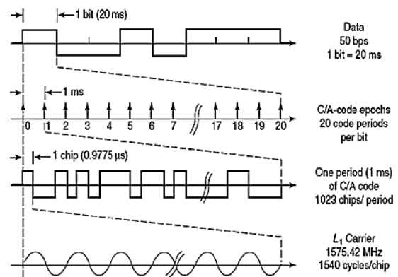
شکل ۴- مراحل تولید سیگنال ارسالی ماهواره
