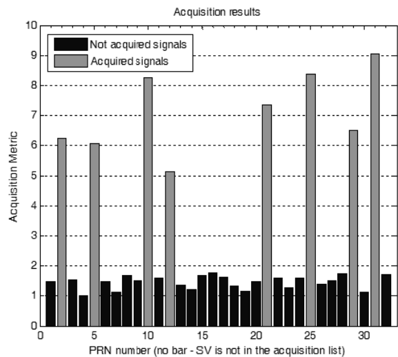
شکل ۱۱- ماهواره‌های در دید گیرنده سافت‌جی‌ان‌اس‌اس با توجه به خروجی Correlation
