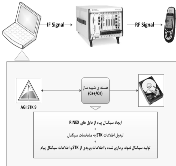
شکل ۸- دیاگرام تولید سیگنال GPS
