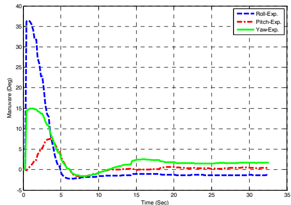
شکل ۷- نمودار زوایای اویلر در راستاهای رول، پیچ و یاو در آزمایش ۲
