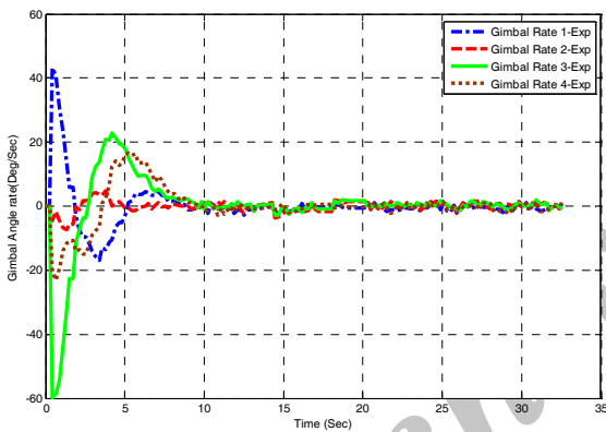
شکل ۹- نمودار نرخ چرخش جیمبال عملگرها در آزمایش ۲
