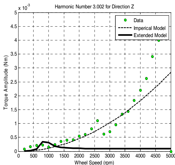
شکل ۳۶- نمودار مربوط به دامنه گشتاور T_z بر حسب سرعت دوران برای عدد هارمونی ۳/۰۰۲
