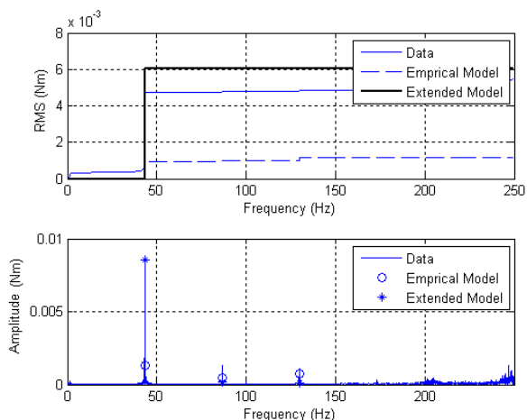
شکل ۳۸- نمودار طیف دامنه و ریشه میانگین مربع تجمعی برای گشتاور T_z در سرعت دوران ۲۶۰۰ دور در دقیقه
