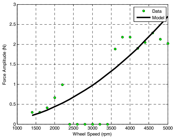
شکل ۶- نمودار دامنه نیرو- سرعت چرخش در هارمونی اول داده‌های F_x پس از حذف اثر مودهای سازهای
