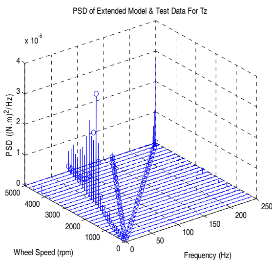
شکل ۳۷- تابع چگالی طیفی (چگالی طیف توانی) داده‌های اندازه‌گیری شده و مدل بسط یافته برای گشتاور T_z
