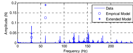
شکل ۲۸- نمودار طیف دامنه و ریشه میانگین مربع تجمعی برای نیروی F_z در سرعت دوران ۱۸۰۰ دور در دقیقه
