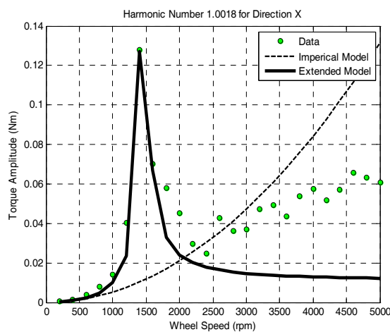
شکل ۲۹- نمودار مربوط به دامنه گشتاور T_x بر حسب سرعت دوران برای عدد هارمونی ۱/۰۰۱۸
