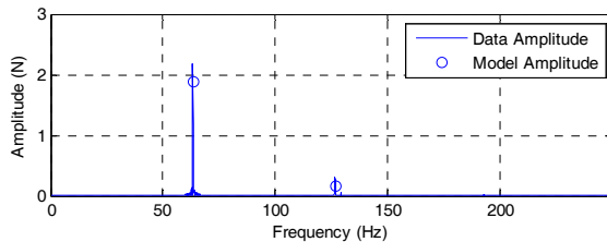
شکل ۸- نمودار ریشه میانگین مربع تجمعی و طیف دامنه برای F_r در سرعت چرخشی ۳۸۰۰ دور در دقیقه
