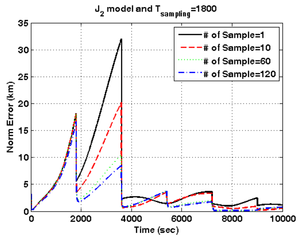
شکل ۱۶- خطای تخمین موقعیت ماهواره نسبت به نرم افزار STK ناشی از تعداد داده در اختیار قرار گرفته، در سر رسیدهای زمانی به فواصل ۱۸۰۰ ثانیه
