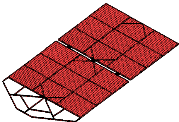
شکل ۱۳- مش‌بندی سازه
