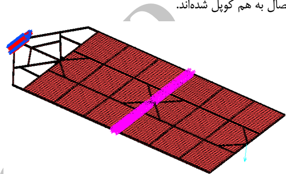
شکل ۱۴- شرایط مرزی و نیروی اعمالی به سازه
