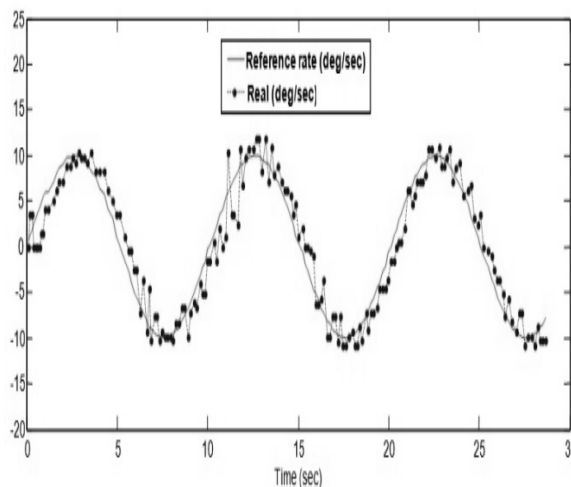
شکل ۴- کنترل نرخ چرخش جیمبال زمانی که نرخ مرجع فرم سینوسی دارد.
