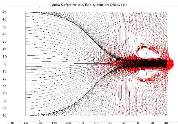
شکل ۸- خطوط جریان در ولتاژ 12 \text{ kV}
