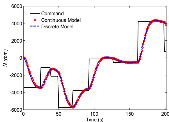
شکل ۲۴- پاسخ سرعت در دو مدل پیوسته و گسسته ARX221
