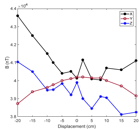
شکل ۸- تغییرات میدان در نقاط با فاصله مشخص از مرکز سیم‌پیچ
