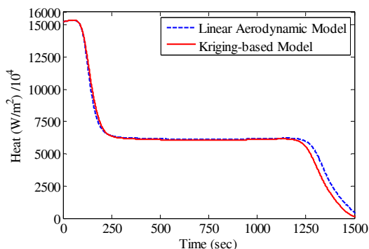
شکل ۹- مقایسه پروفیل شار حرارتی بر حسب زمان
