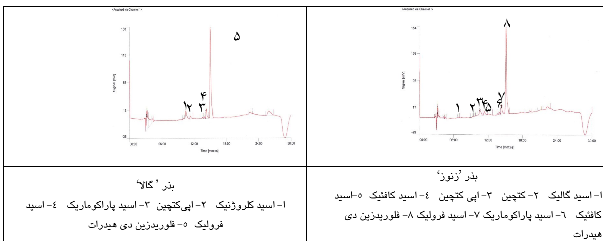
شکل ۳- کروماتوگرام عصاره‌های بذر ارقام سیب 'گالا' و 'زنوز' با استفاده از فاز متحرک: ۲٪ اسیتک اسید در متانول و آب برای جداسازی ترکیبات پلی فنلی و فلاونوئیدی
