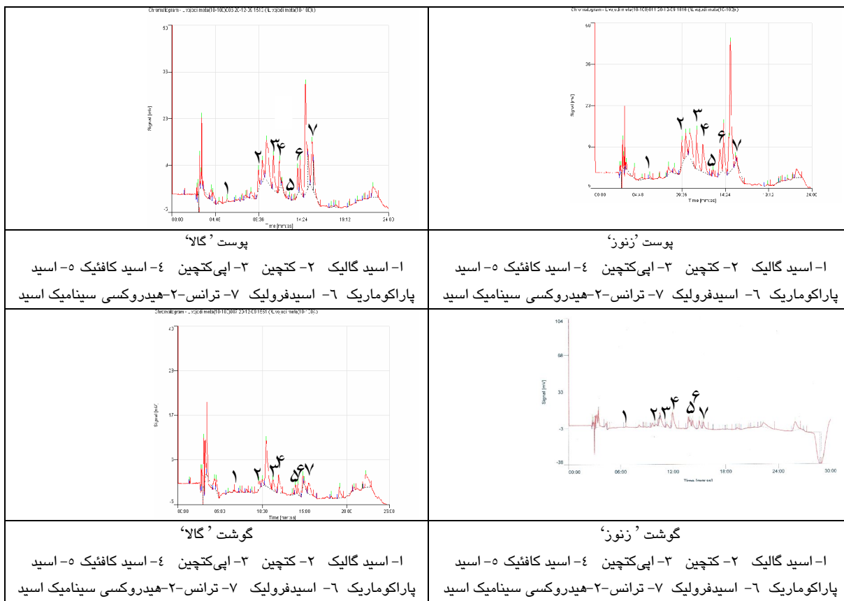
شکل ۲- کروماتوگرام عصاره‌های گوشت و پوست ارقام سیب 'گالا' و 'زنوز' با استفاده از فاز متحرک: ۲٪ اسیتک اسید در متانول و آب برای جداسازی ترکیبات پلی فنلی و فلاونوئیدی.
