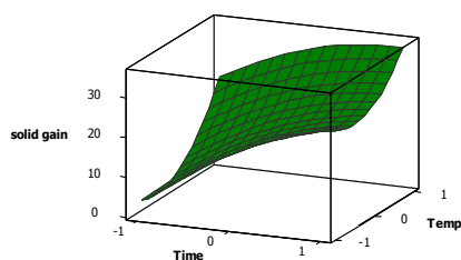
شکل ۳- نمودار خطی و سطحی جذب ساکارز (%) در برابر زمان (ساعت) و دما (درجه سانتی‌گراد) (در غلظت ۵۰٪ و فرکانس ۳۵ کیلوهرتز)
