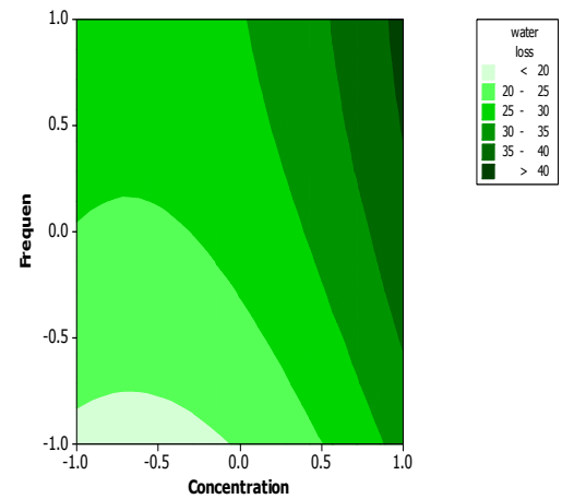
شکل ۲- نمودار خطی و سطحی از دست دادن آب (%) در برابر فرکانس (کیلوهرتز) و غلظت (%) (در دمای ۵۰ درجه سانتی‌گراد و زمان ۷ ساعت)
