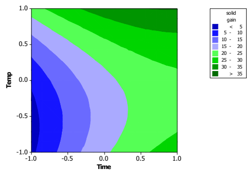
شکل ۳- نمودار خطی و سطحی جذب ساکارز (%) در برابر زمان (ساعت) و دما (درجه سانتی‌گراد) (در غلظت ۵۰٪ و فرکانس ۳۵ کیلوهرتز)
