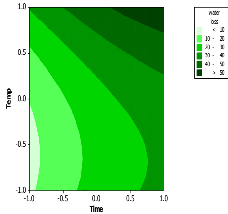
شکل ۱- نمودار خطی و سطحی از دست دادن آب (%) در برابر زمان (ساعت) و دما (درجه سانتی‌گراد) (در فرکانس ۳۵ کیلوهرتز، غلظت ۵۰٪)
