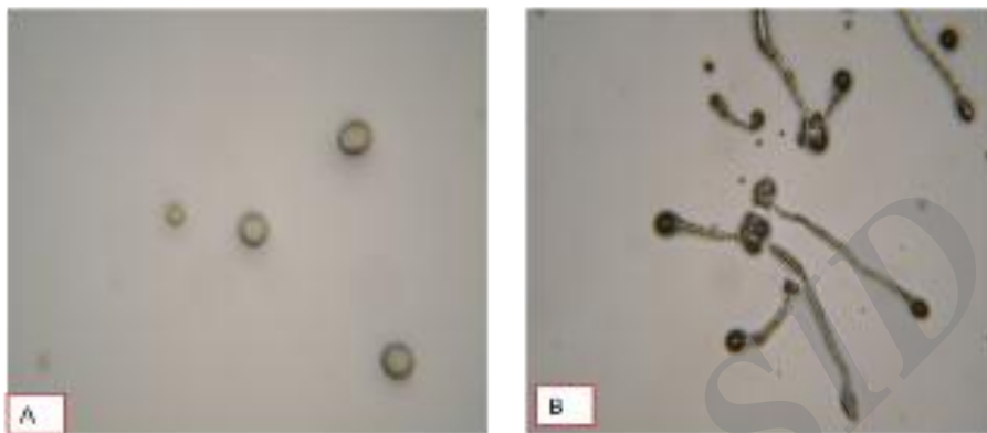
شکل ۳. اشکال میکروسکوپی دانه‌های گرده (A) دانه‌گرده رقم قزل‌اوزوم؛ (B) دانه‌گرده بی‌دانه سفید (شاهد).
