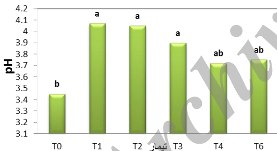
شکل ۱. مقایسه میانگین اثر تیمار بر pH عصارة رقم قزل‌اوزوم
