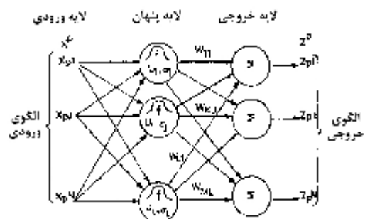
شکل 2- تصویر شماتیک شبکه RBF
