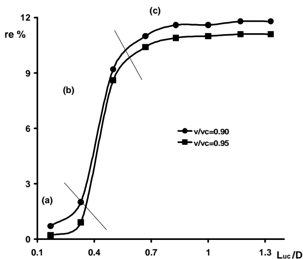
شکل 7- تغییرات درصد کاهش عمق آبشستگی با طول بی بعد طوق در بالادست.
