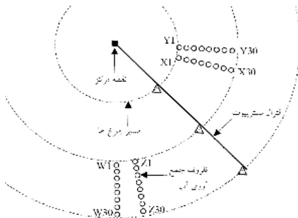
شکل 3- موقعیت قرارگیری ردیف‌های ظروف جمع آوری آب سیستم ستریپت
