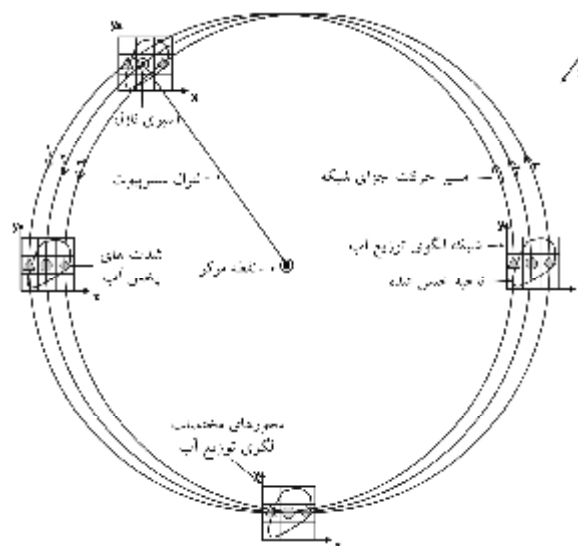
شکل 1- شبکه دینامیک و مسیر حرکت شماتیک اجزای الگوی توزیع اسپری نازل منفرد
