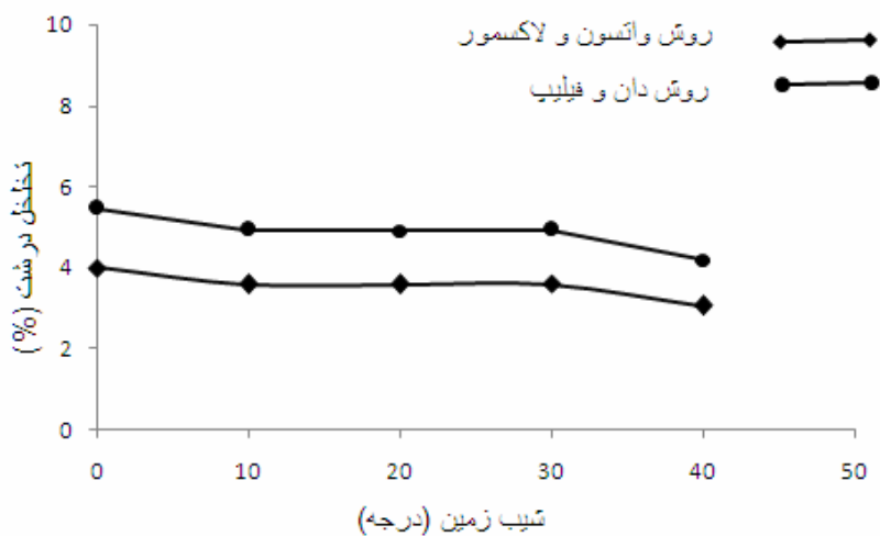
شکل 2- تغییرات مقدار تخلخل درشت با تغییرات شیب زمین
