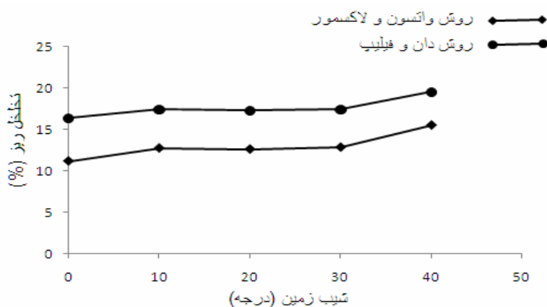
شکل 4- تغییرات مقدار تخلخل ریز با تغییرات شیب زمین
