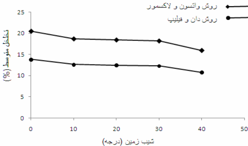
شکل 3- تغییرات مقدار تخلخل متوسط با تغییرات شیب زمین
