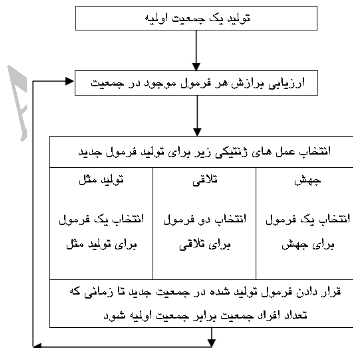
شکل 2- طرح کلی گام‌های اجرایی برنامه‌ریزی ژنتیک
