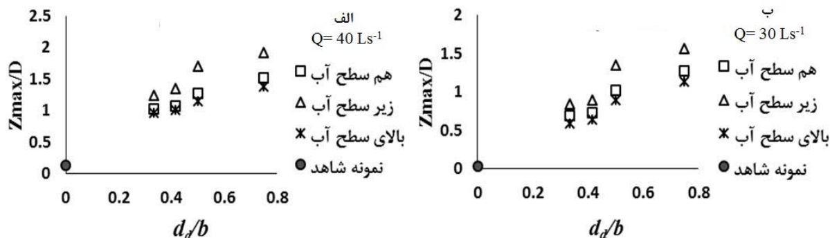
شکل ۱۲- بیشینه عمق آبستگي در مقابل نسبت عرض اجسام شناور چوبی به عرض کانال برای الف) Q=40 L s^{-1} و ب) Q=30 L s^{-1} .
