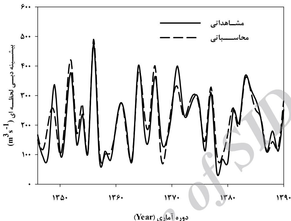
شکل ۹- نتایج مدل‌سازی مدل ARMA(1,0) در مدل‌سازی داده‌های بیشینه دبی لحظه‌ای رودخانه سیمینه رود در دوره آماری ۱۳۴۶-۱۳۹۰.
