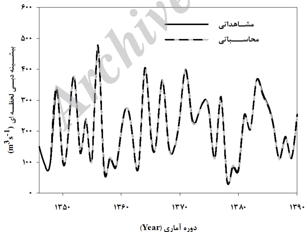
شکل ۸- نتایج مدل‌سازی مدل AR-PARCH در مدل‌سازی داده‌های بیشینه دبی لحظه‌ای رودخانه سیمینه‌رود در دوره آماری ۱۳۴۶-۱۳۹۰.
