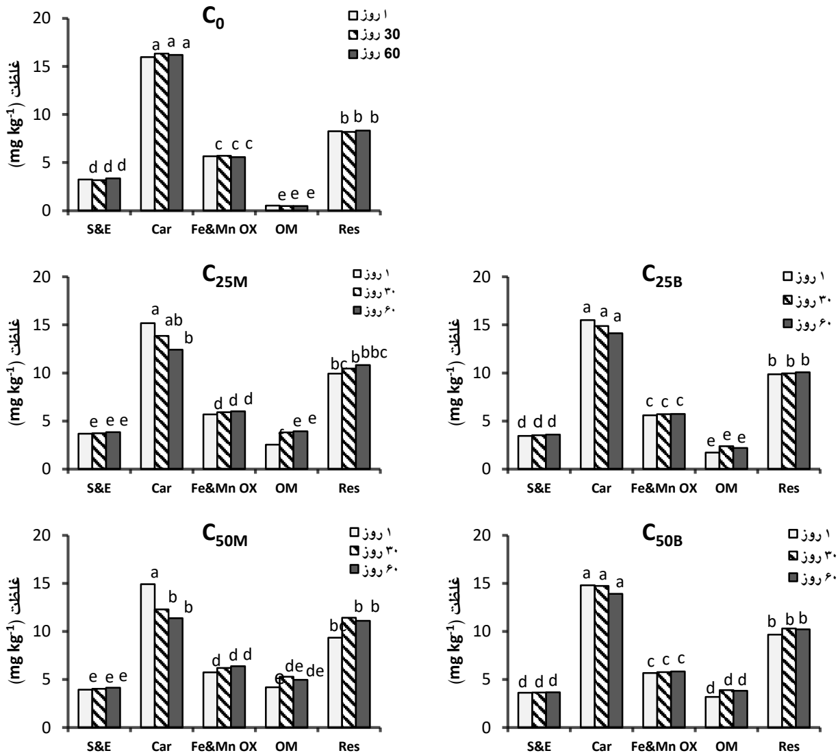
شکل ۱- تغییرات شکل‌های شیمیایی کادمیم (S&E: محلول و تبادلی؛ Car: کربناتی؛ Fe&Mn OX: اکسیدهای آهن و منگنز؛ OM: مواد آلی؛ Res: باقی‌مانده) در زمان‌های خواباندن مختلف برای تیمارهای C 0 : شاهد، C 25B : خاک تیمار شده با ۲۵ تن در هکتار کمپوست بقایای نیشکر، C 50B : خاک تیمار شده با ۵۰ تن در هکتار کمپوست بقایای نیشکر، C 25M : خاک تیمار شده با ۲۵ تن در هکتار کود گاوی و C 50M : خاک تیمار شده با ۵۰ تن در هکتار کمپوست بقایای نیشکر.
