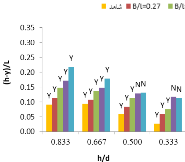
شکل ۹- تغییرات گرادیان جریان خروجی به ازای عمق
