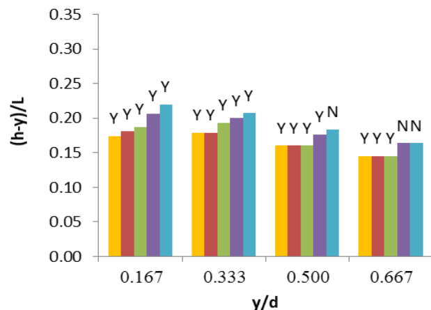
شکل ۸- تغییرات گرادیان جریان خروجی به ازای عمق نسبی آب کانال و فاصله نسبی صفحه‌های مشبک ( B/l ) در شرایط صعود سطح ایستابی.
