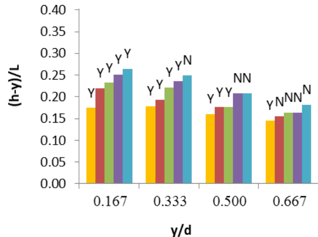
شکل ۸- تغییرات گرادیان جریان خروجی به ازای عمق
