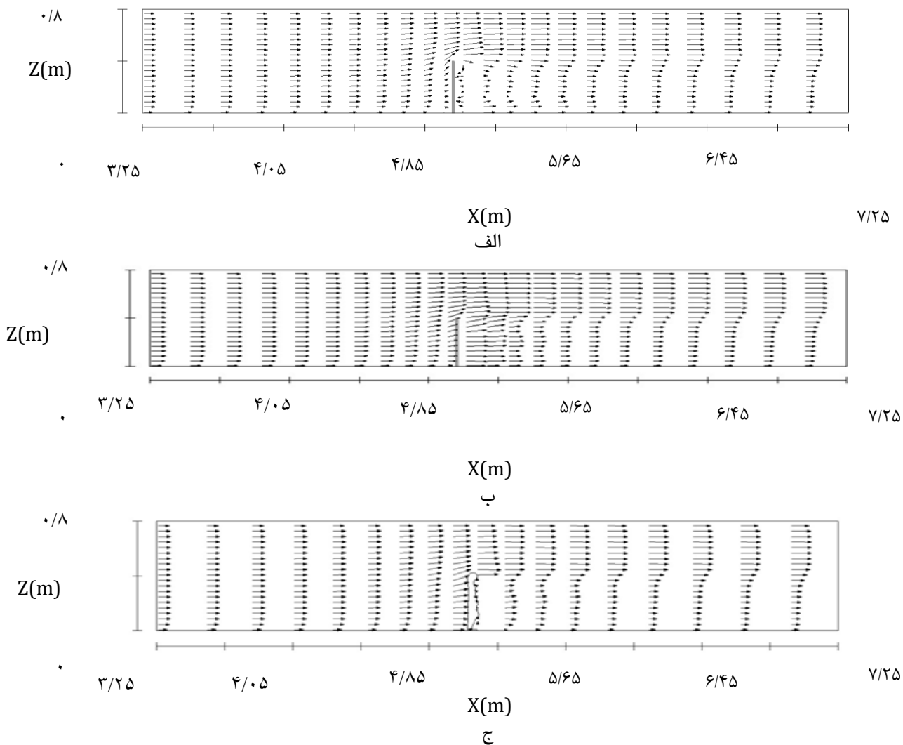
شکل ۴- بردارهای سرعت در مجاورت آبشکن با طول ۰/۴ متر به ترتیب در فاصله‌های الف ( Z=0.09\text{cm} ) ب ( Z=0.15\text{cm} ) ج ( Z=0.2\text{cm} )
